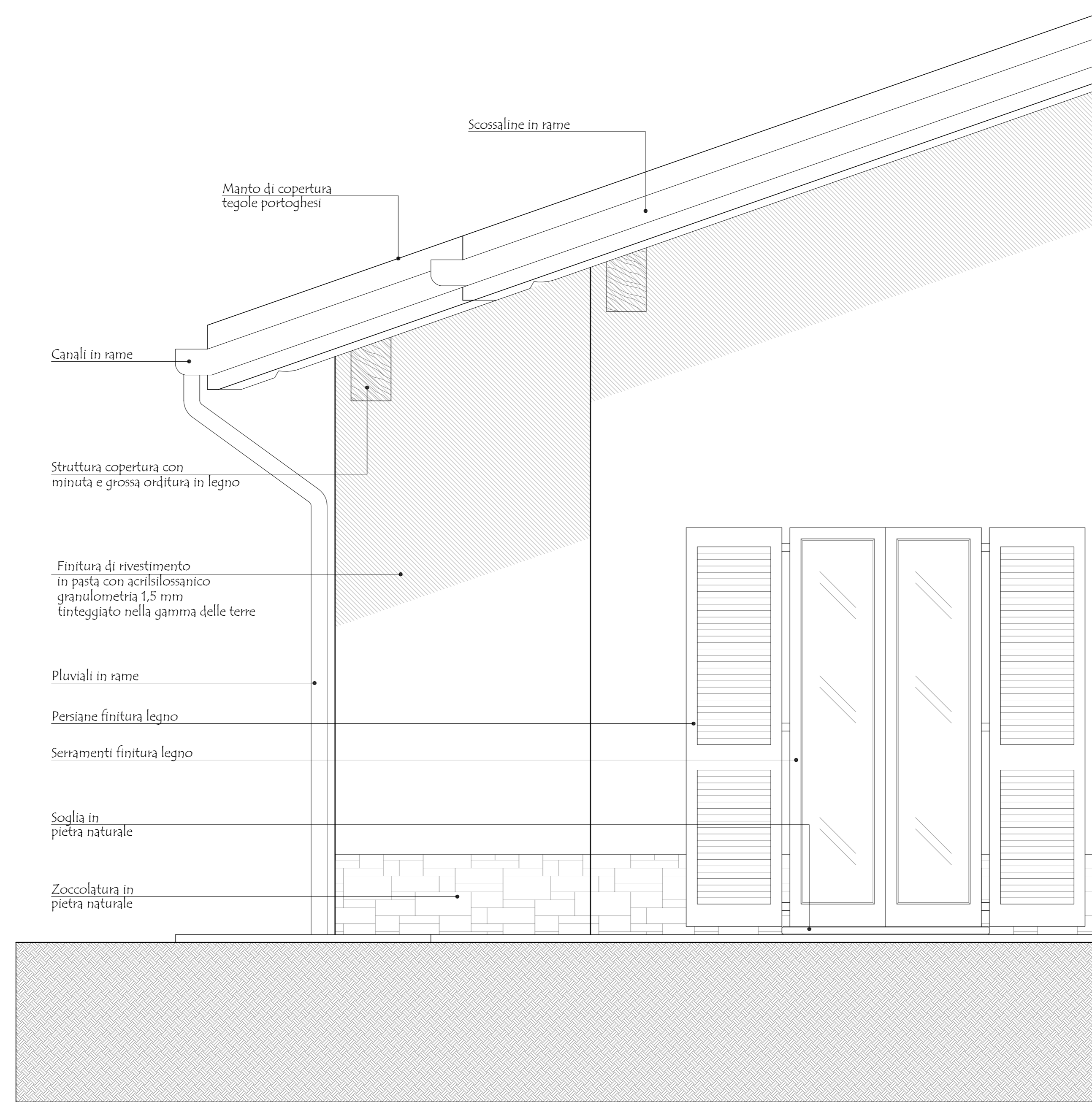
PARTICOLARE PROSPETTO
