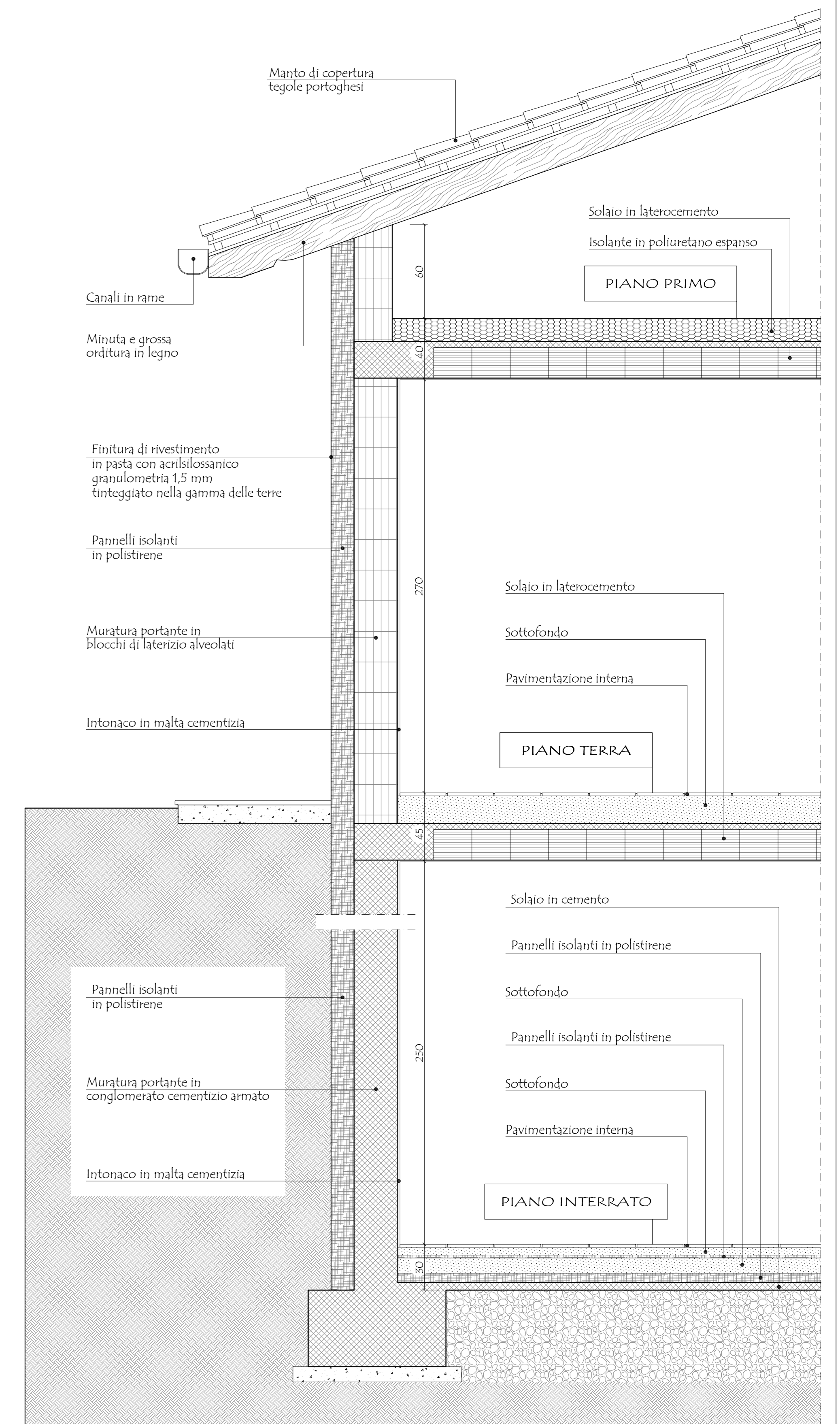
PARTICOLARE SEZIONE
