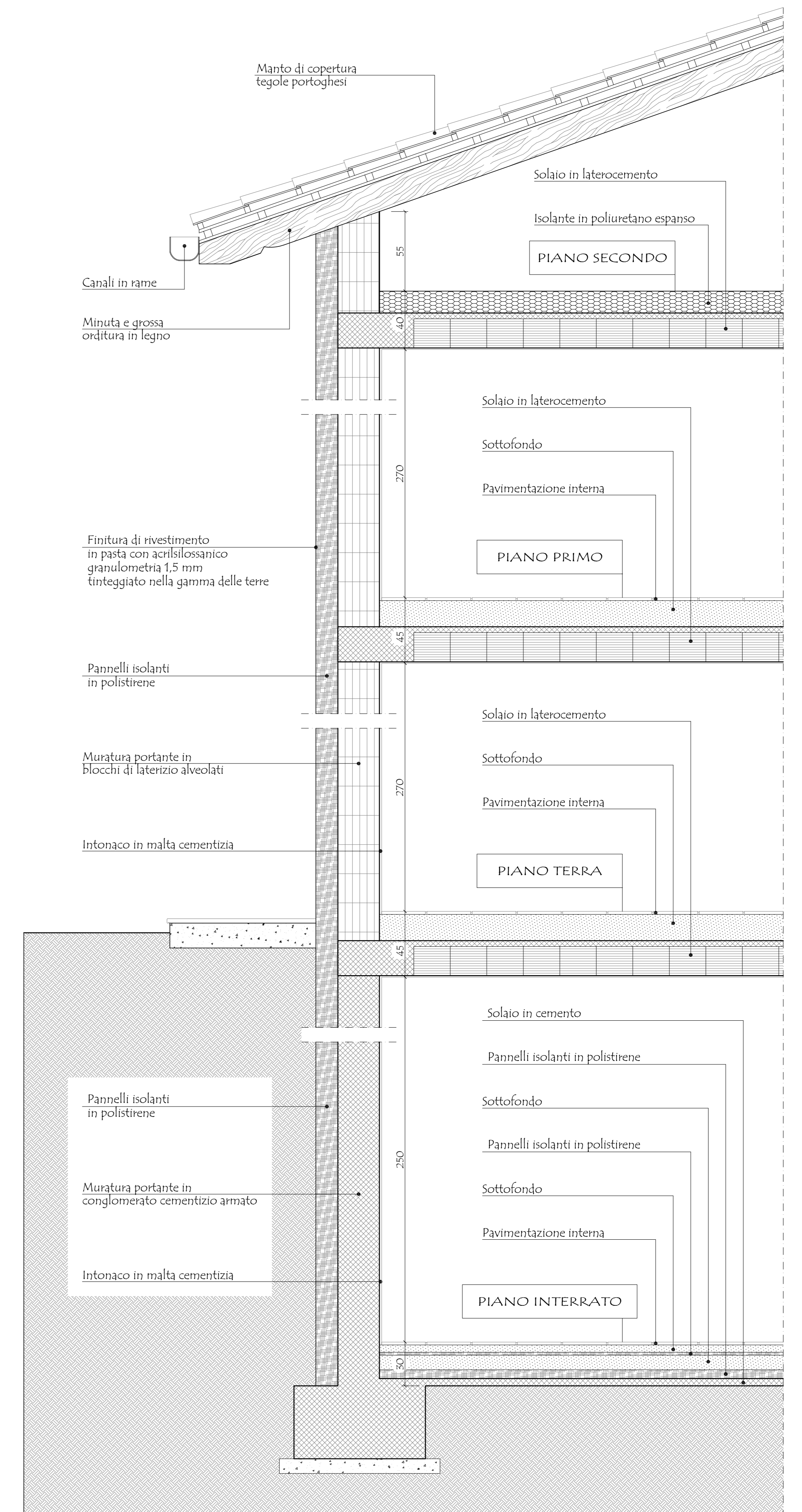
PARTICOLARE SEZIONE
