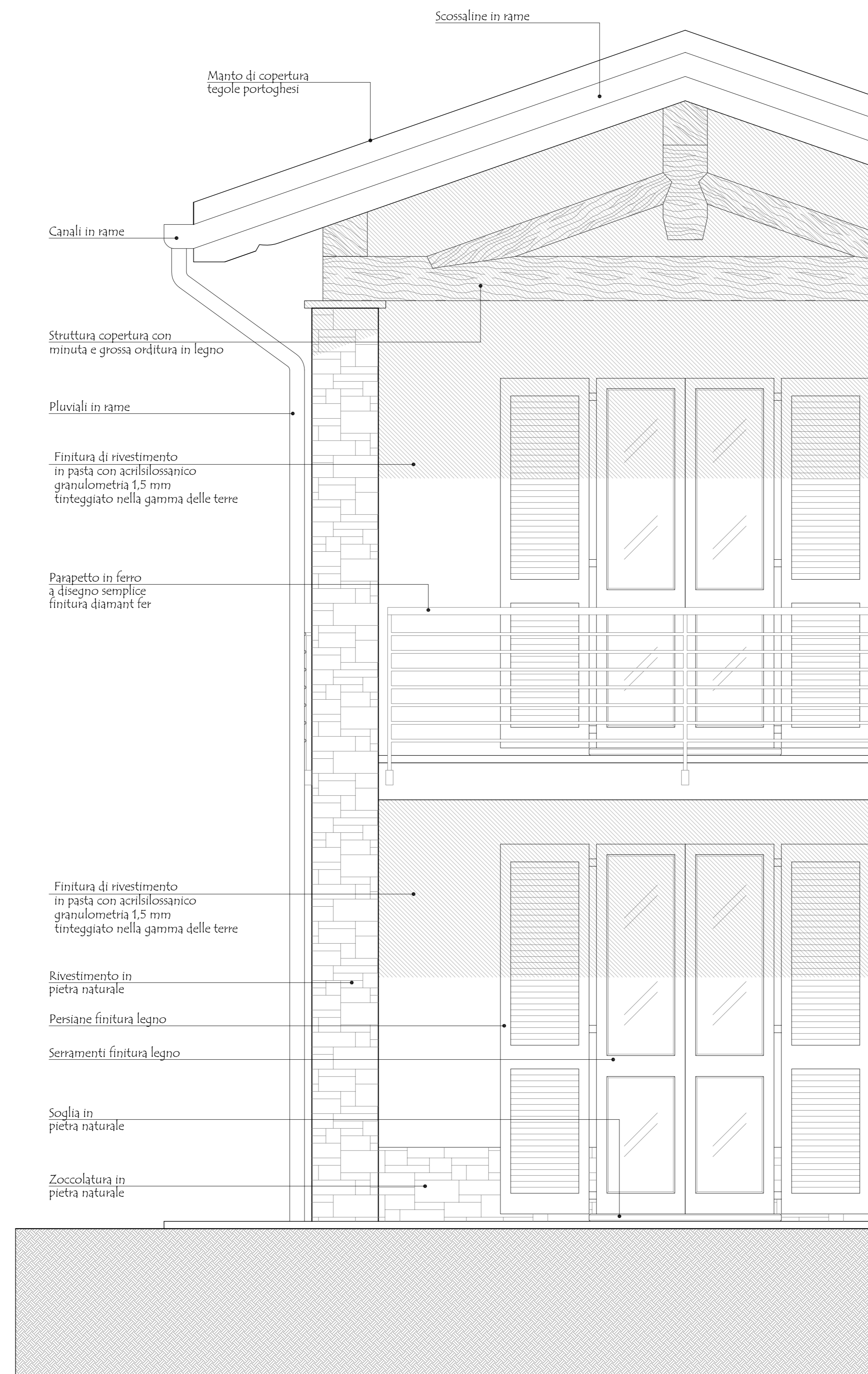
PARTICOLARE PROSPETTO
