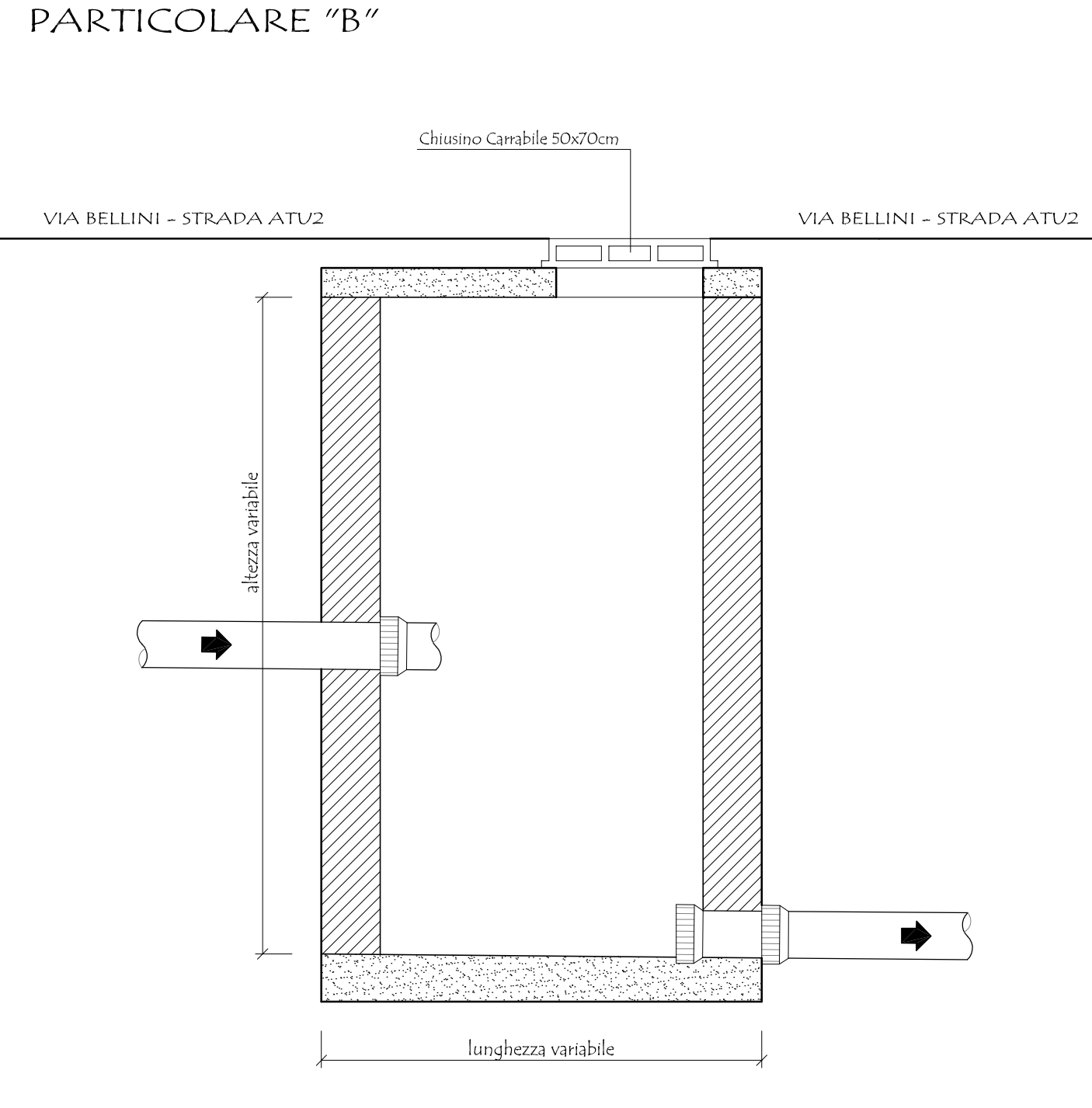
PARTICOLARE CAMERETTA FOGNATURA VIA BELLINI - STRADA ATU2 - SCALA 1:20
