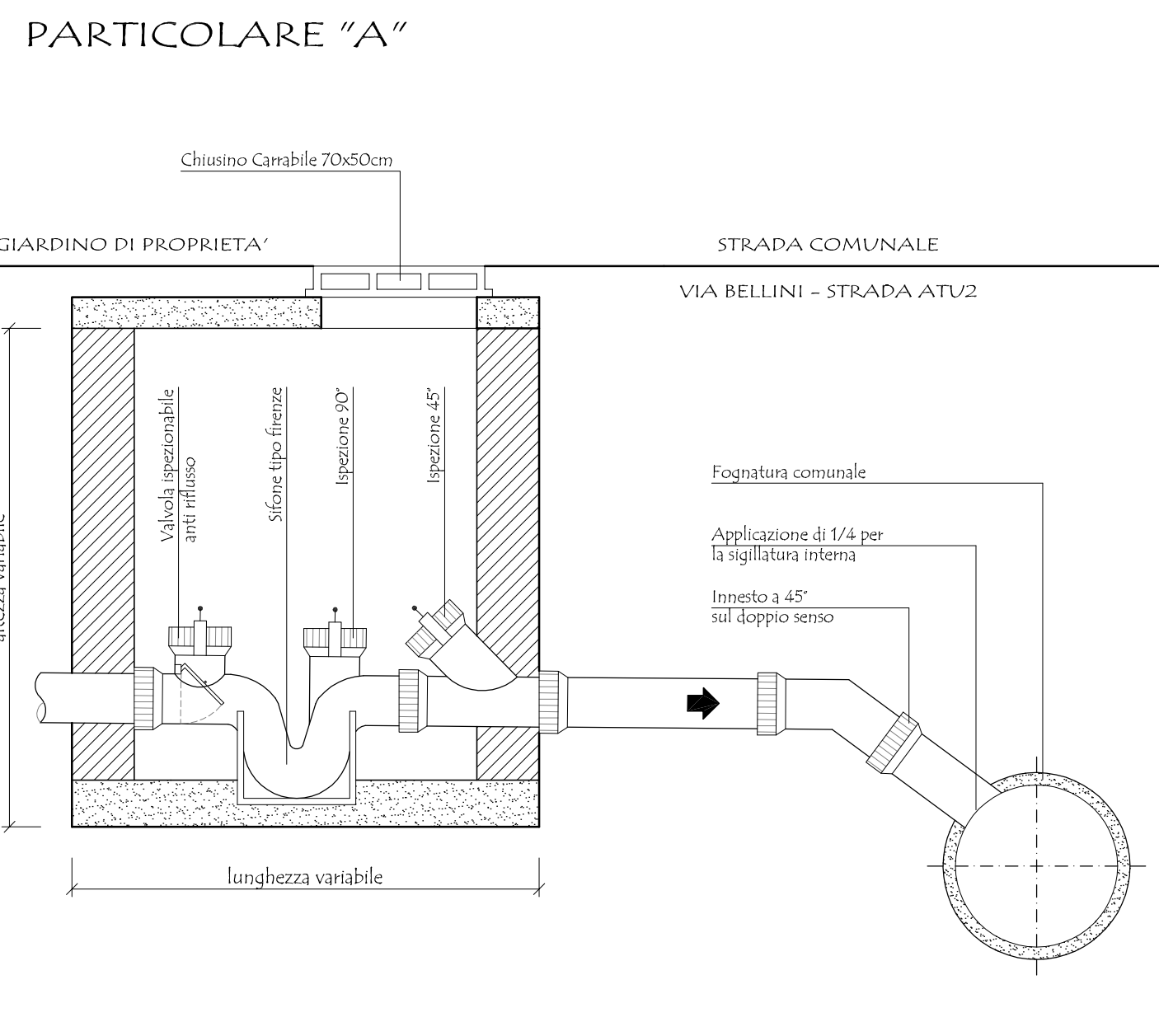
PARTICOLARE BRAGA-SIFONE-ISPEZIONE VIA BELLINI - STRADA ATU2 - SCALA 1:20
